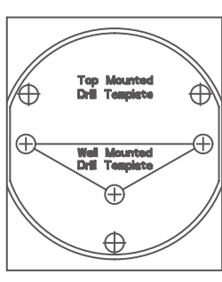
Vrtací šablona (1×)
